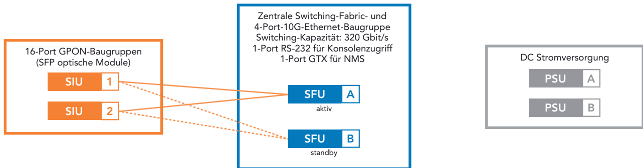
Abbildung 1: Redundante Systemarchitektur
