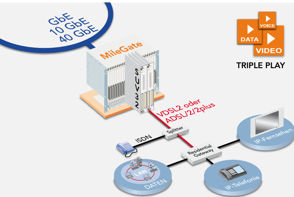
Zwei MileGate SUV32 für bis zu 192 mit Vectoring erweiterte VDSL2-Anschlüsse
